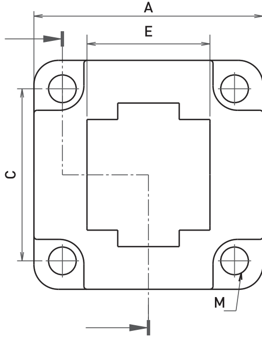
EBX YER BAĞLANTI ( ISO ,VDMA )
